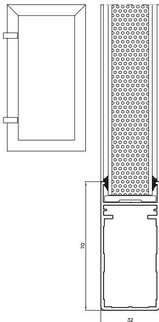
Przekrój pionowy skrzydła okiennicy panelowej
