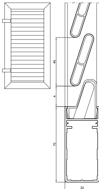
Przekrój pionowy skrzydła okiennicy lamelowej
